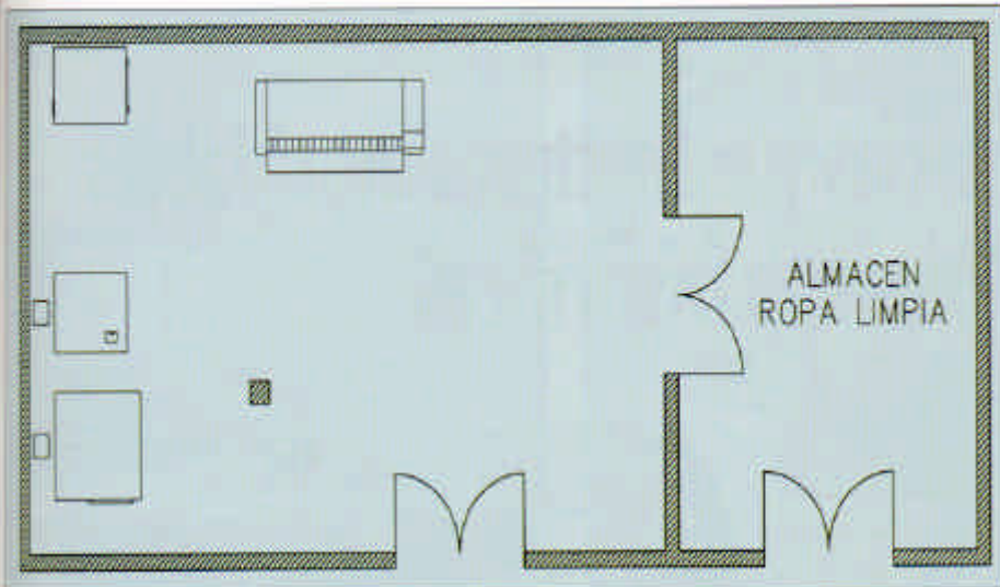
Plano de la instalación, que incluye dos lavadoras centrifugadoras, una secadora, una planchadora-secadora y carros para el transporte de ropa.
